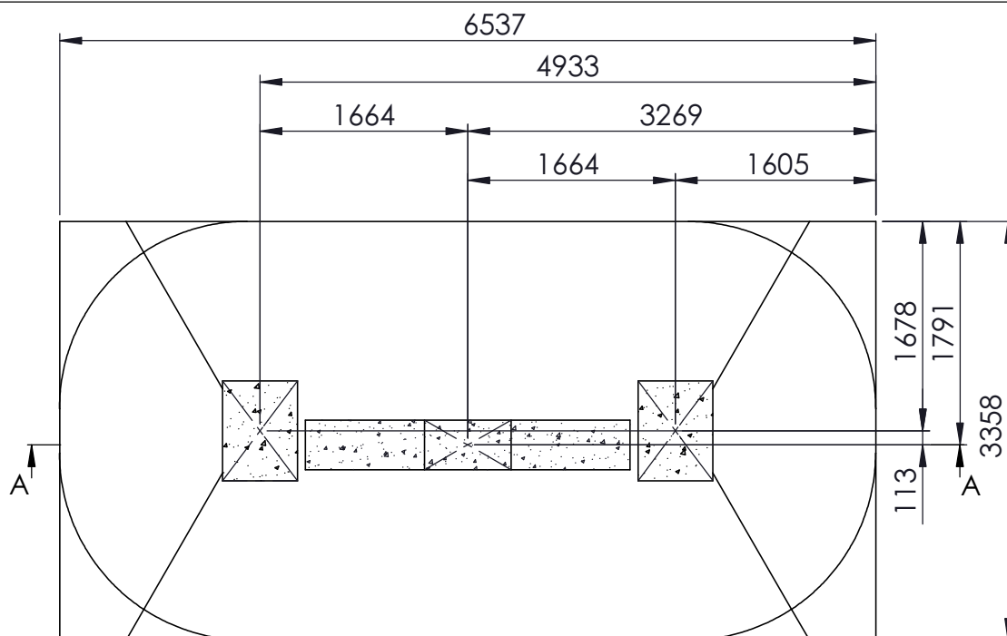
SECTION A-A SCALE 1 : 55
