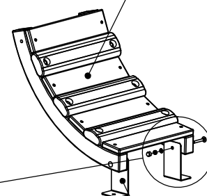
F300-M-Voetijzer-01 2x
